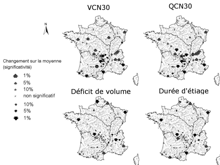
Figure 3 : Tendances détectées sur les variables d'étiage (voir définitions page suivante).
