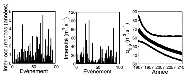
Figure 4 : (a) série des intervalles inter-occurrences, (b) série des intensités, (c) trajectoire de la crue décennale au cours du temps, et intervalle de confiance à 90 %.
