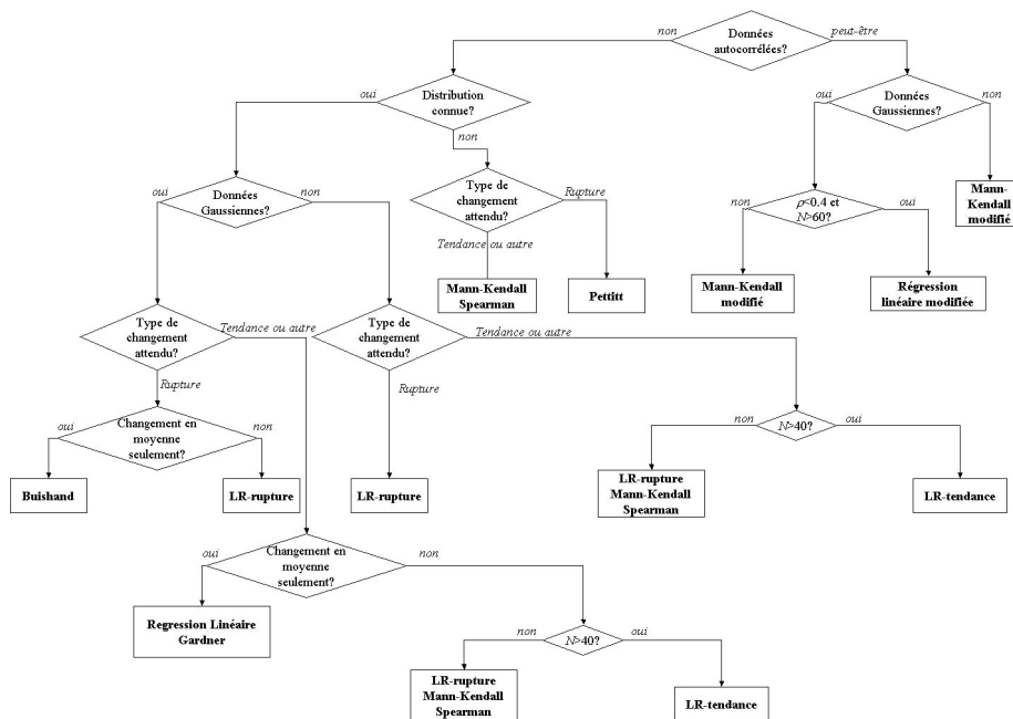
Figure 1 : Schéma de sélection d'un test de stationnarité adapté aux caractéristiques probabilistes de la variable étudiée.
