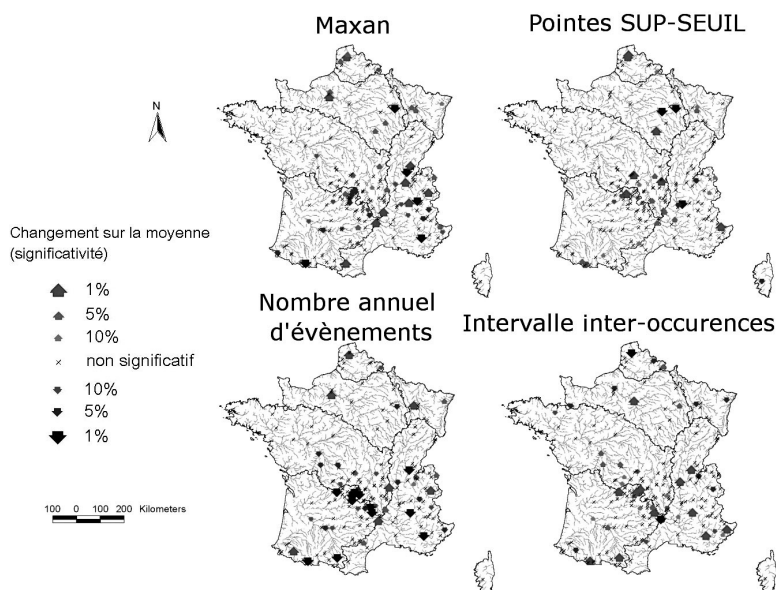
Figure 2 : Tendances détectées sur les variables de crue (voir définitions page suivante).
