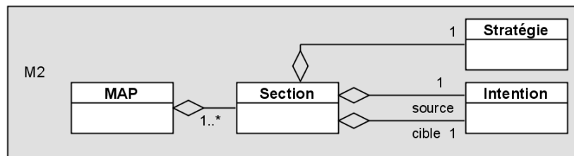
Figure 15. Extrait du méta-modèle de processus orienté stratégie MAP.
