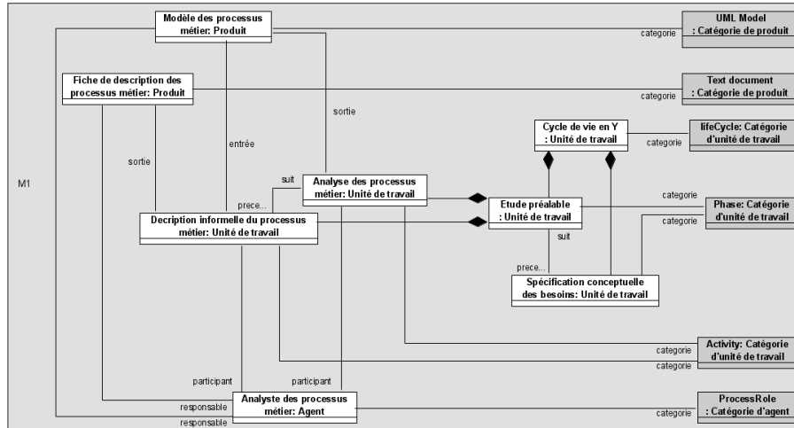
Figure 23. Construction d'une partie de SPEM et de Symphony avec le méta-modèle de processus.
