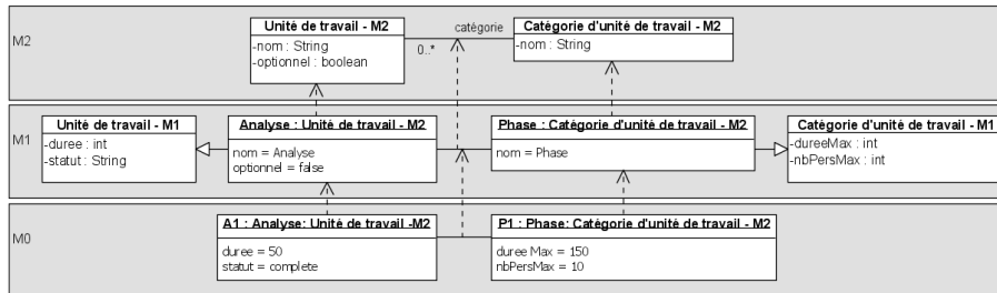
Figure 19. Instanciation et héritage d'attributs de méta-classes.
