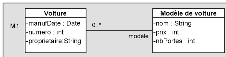
Figure 18. Imitation du patron « Item-Description ».
