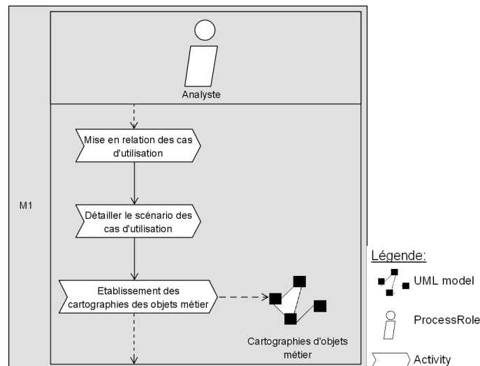
Figure 2. Extrait du modèle de processus orienté activité Symphony.
