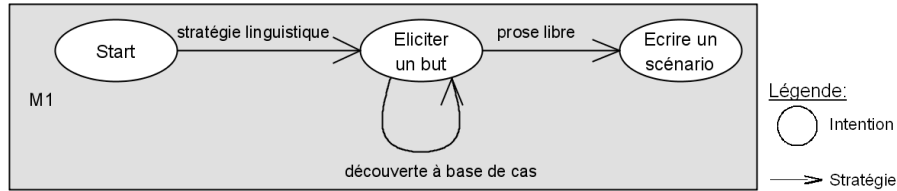
Figure 14. Extrait du modèle de processus orienté stratégie, CREWS- l'Écritoire dans le formalisme MAP.
