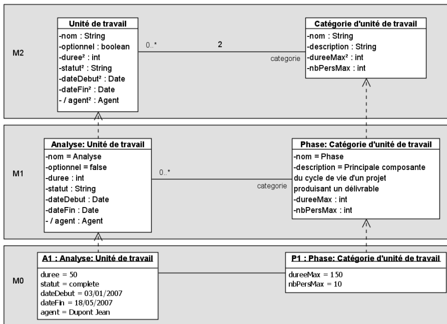
Figure 20. Utilisation de l'instanciation profonde pour la méta-modélisation de processus.
