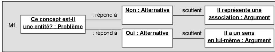
Figure 10. Extrait d'un modèle de processus orienté décision comme instance du méta-modèle de (Potts et al.).
