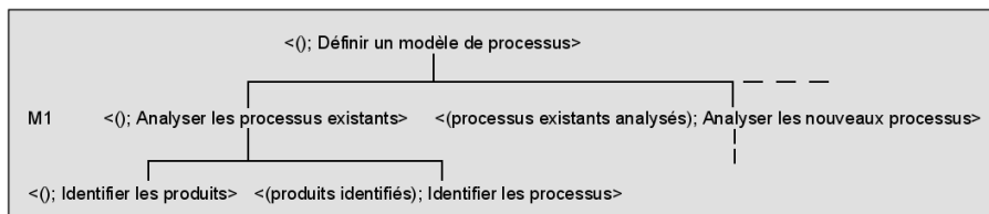
Figure 11. Extrait d'un modèle de processus orienté contexte, dans le formalisme NATURE.
