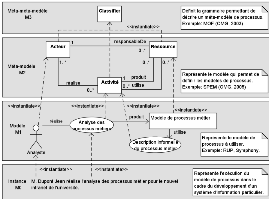
Figure 1. Exemple d'architecture à quatre niveaux pour les processus.
