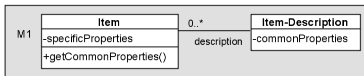
Figure 17. Le patron « Item-Description ».
