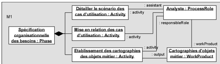
Figure 4. Extrait du modèle de processus orienté activité Symphony comme instance de SPEM.
