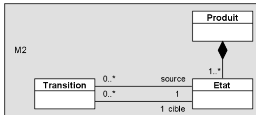
Figure 6. Extrait du méta-modèle du State-Transition.
