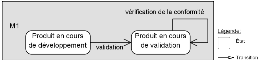
Figure 5. Extrait d'un modèle de processus orienté produit représenté avec le formalisme des diagrammes états-transitions d'UML.
