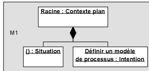
Figure 13. Extrait d'un modèle de processus orienté contexte comme instance de NATURE.
