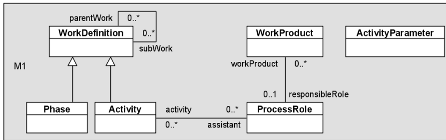
Figure 3. Extrait du méta-modèle SPEM.
