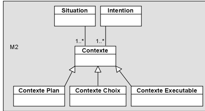
Figure 12. Extrait du méta-modèle de processus orienté contexte NATURE.
