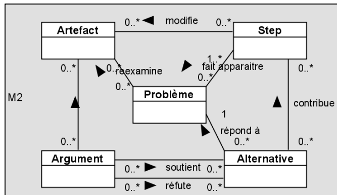
Figure 9. Méta-modèle de processus orienté décision de Potts et al.
