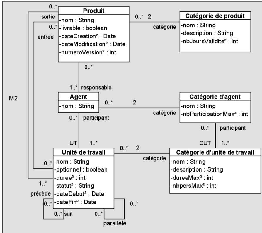
Figure 22. Extrait d'un méta-modèle de processus : trois imitations du patron « Concept – Catégorie de Concept ».
