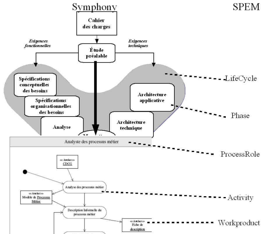
Figure 21. Illustration des catégories de concepts de SPEM et des concepts de Symphony.
