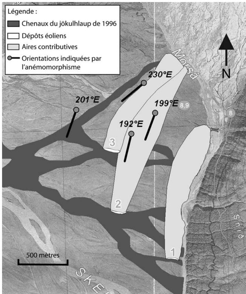
Figure 6 : Cartographie des orientations indiquées par l'anémomorphisme et des limites des aires contributives
