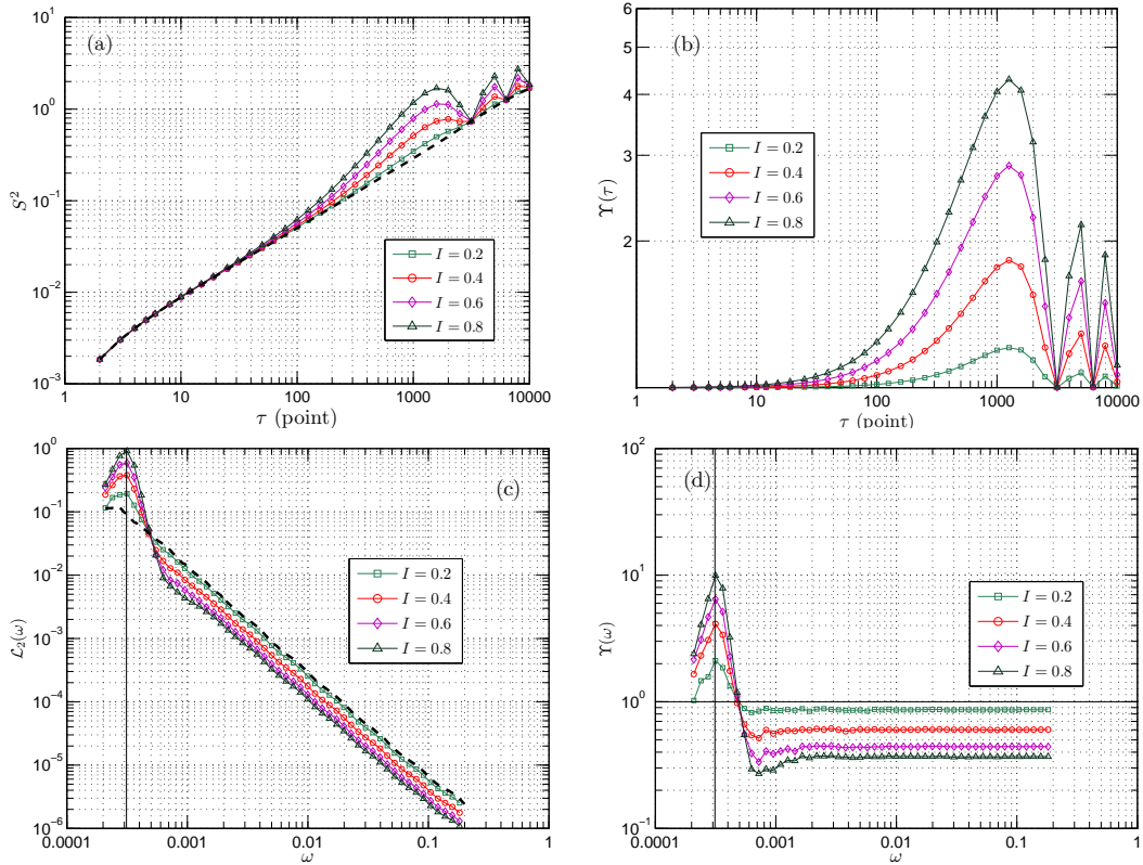
Fig. 8. Représentation de l'effet périodique, (a) fonction de structure d'ordre 2, (b) le ratio \Upsilon(\tau) , (c) spectre de Hilbert \mathcal{L}_2(\omega) , (d) le ratio \Upsilon(\omega) , où f = 1/3200 et l'intensité I = 0.2 ( \square ), 0.4 ( \circ ), 0.6 ( \diamond ) and 0.8 ( \triangle ).
