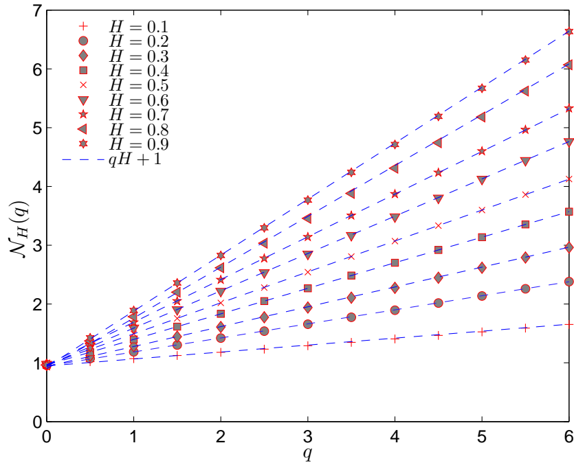
Fig. 5. Représentation des exposants N(q) en fonction de q , où H varie de 0.1 à 0.9. Les valeurs obtenues sont comparées aux expressions théoriques 1 + qH , montrant une parfaite adéquation.
