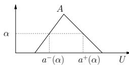
Fig. 10. Input notation
