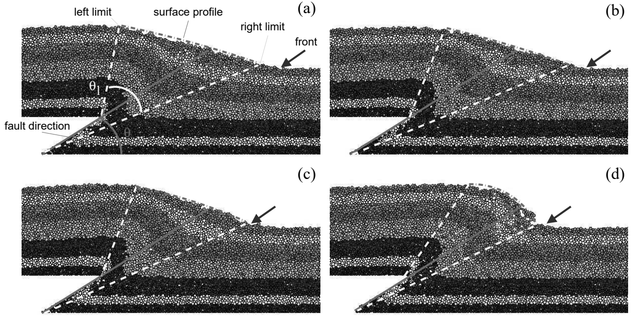
Figure 12. Free surface profiles for different values of \gamma : (a) 0\text{ N} , (b) 10^3\text{ N} , (c) 10^4\text{ N} and (d) 10^5\text{ N}
