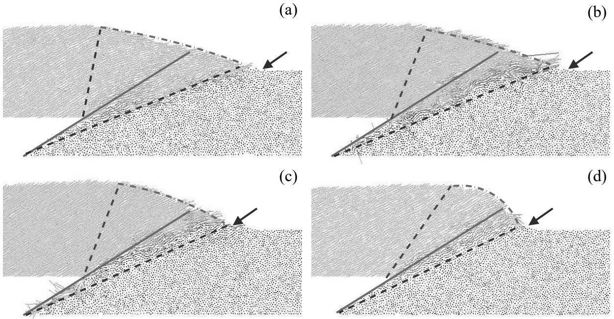
Figure 13. Velocity fields for different values of \gamma : (a) 0\text{ N} , (b) 10^3\text{ N} , (c) 10^4\text{ N} and (d) 10^5\text{ N}
