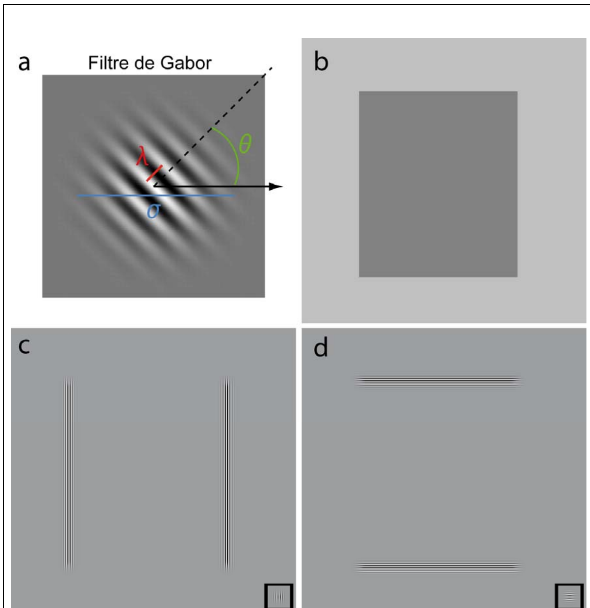
Figure E2 : Exemple simple d'une des utilisations des filtres de Gabor en analyse d'images. (a) Image d'un filtre de Gabor et ses paramètres associés. (b) L'objet dont on veut détecter les bords est un carré gris sur un fond plus clair. En convoluant cette image avec les filtres de Gabor avec \theta=0^\circ et \theta=90^\circ ( \lambda=4 pixels, \sigma=8 pixels), on obtient les images données en (c) et (d). Les filtres de Gabor utilisés sont montrés en insert.
