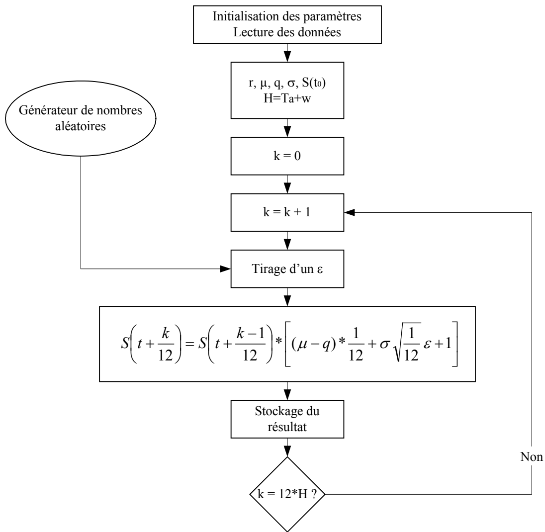
Figure 2 : Schéma de génération des trajectoires du cours de l'action
