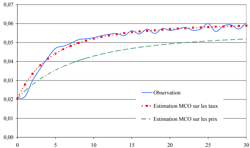
Fig. 4. Taux instantanés espérés en fonction de leur échéance et de la technique d'estimation des paramètres
