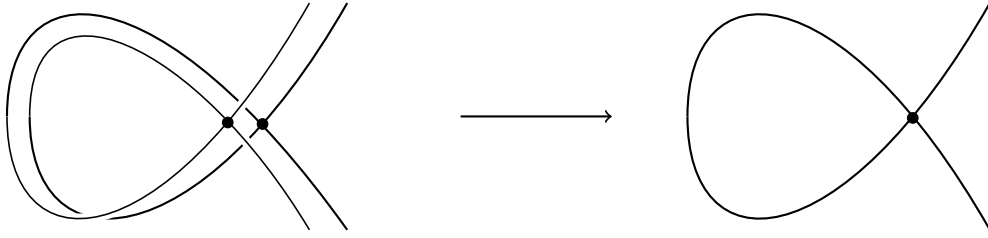
FIG. 1 – Revêtement double de la cubique nodale
