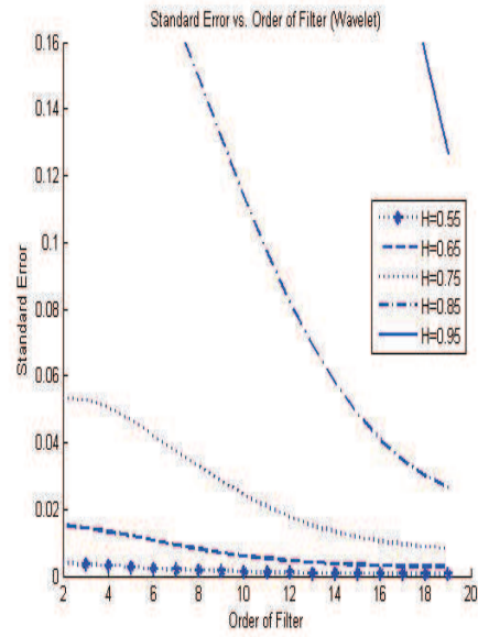
Fig. 2.: Wavelet Filters.
