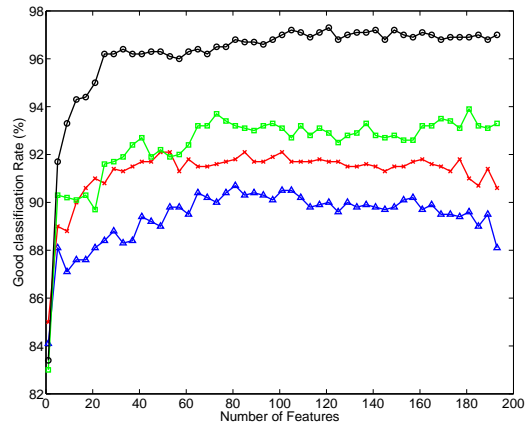
(b) JPHS
