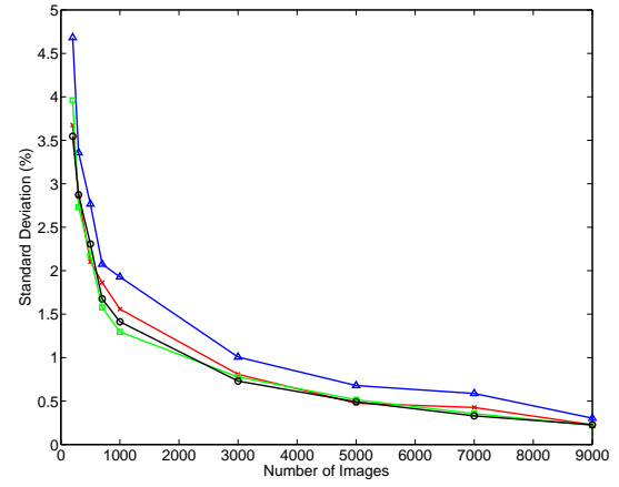
(d) MM3
