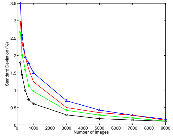
(b) JPHS
