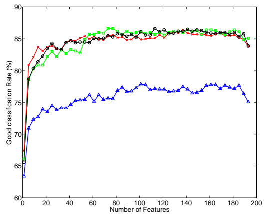
(d) MM3
