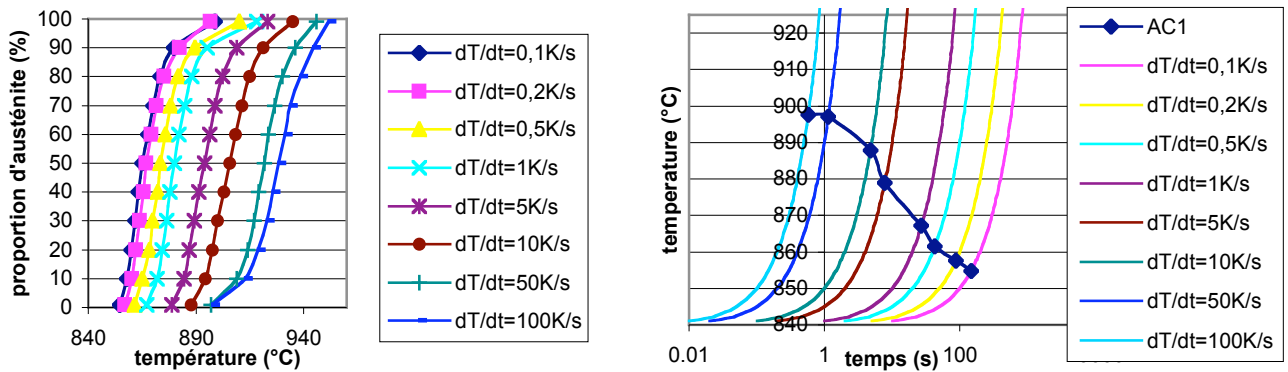
Figure 2a. Cinétique de transformation austénitique y(T) . Figure 2b. Courbe de début de transformation A_S (ou A_{C1} ). Acier T91 (X10CrMoVNb9-1) –microstructure initiale de type martensite revenue–, d'après Duthilleul et Brachet (2005).
