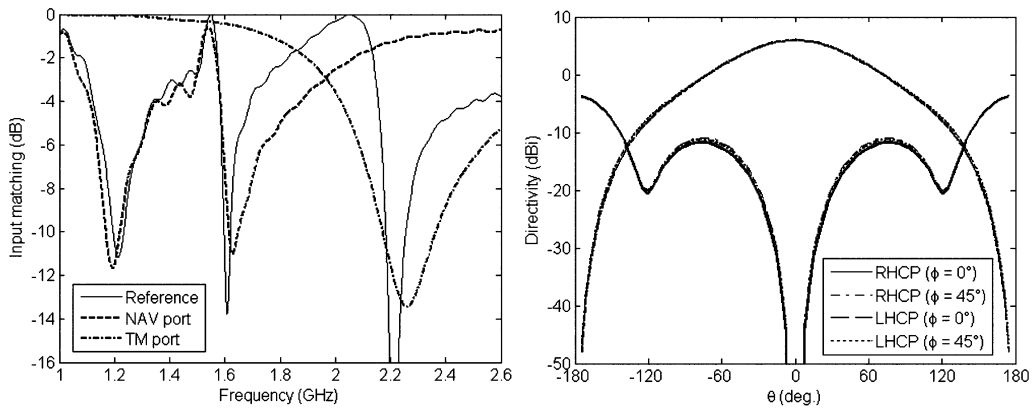
Fig. 2: Input matching
