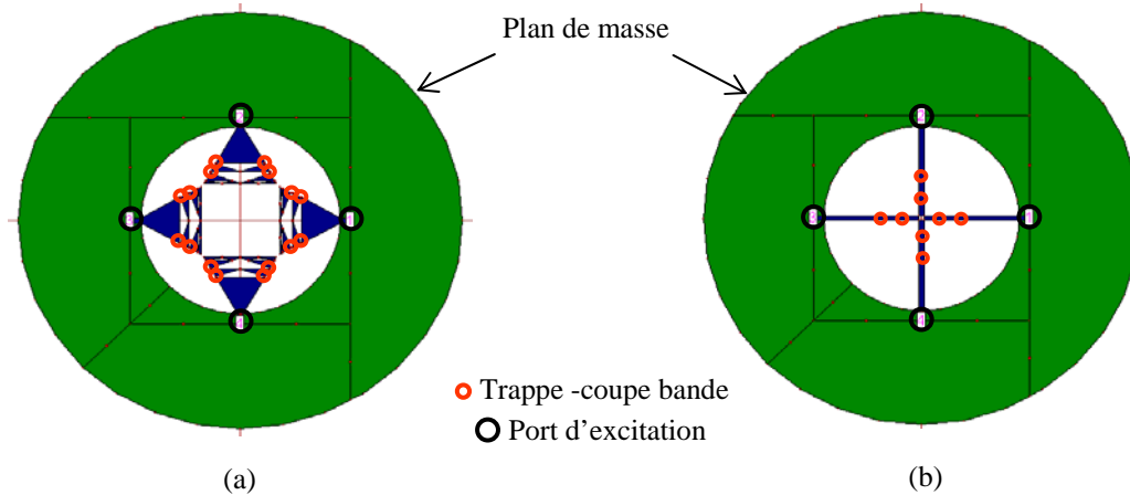
Figure 2 : Antennes tri-bandes à trappes à base : (a) de triangles de Sierpinski et (b) d'éléments filaires
