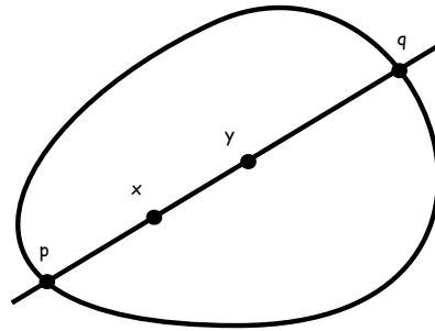
FIGURE 1. La distance de Hilbert
