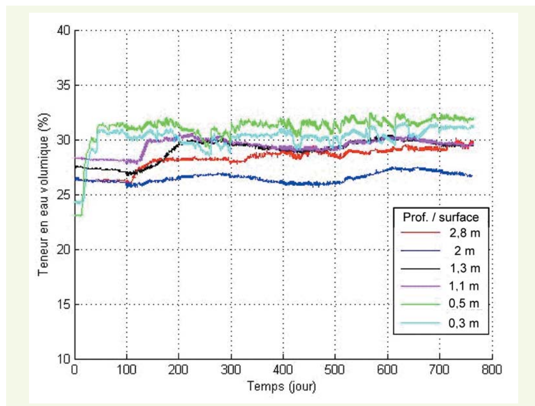
figure 14 Fluctuations temporelles de la teneur en eau volumique dans un remblai en limon sableux à différentes profondeurs.
