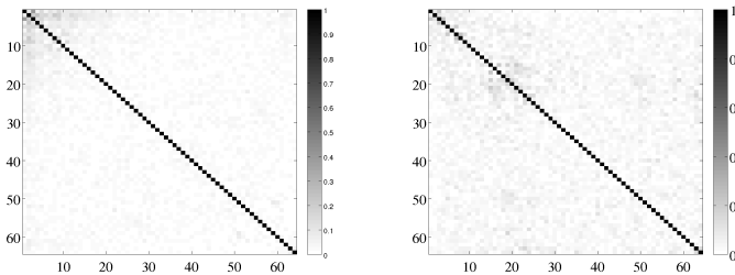
FIGURE 1 – Matrices de corrélation des \{a_t\} estimés par CEM : parties non-transitoires (gauche) et transitoires (droite)
