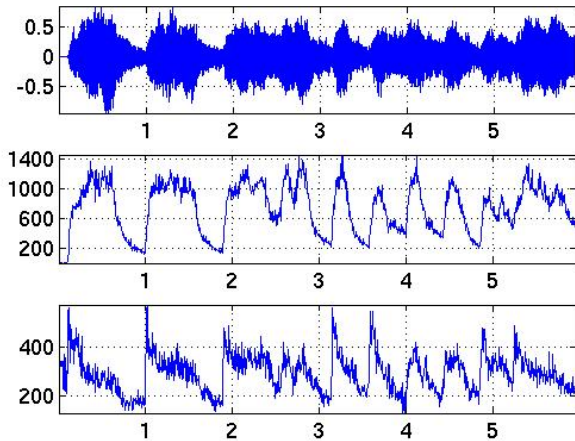
FIGURE 3 – Signal d’orgue (haut), et indices Z_p (milieu) et Z_p^{(n)} (bas)
