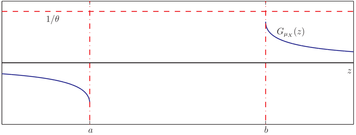
(b) When 1/\theta > G_{\mu_X}(b) , \lambda_1(X + P) \rightarrow b .
