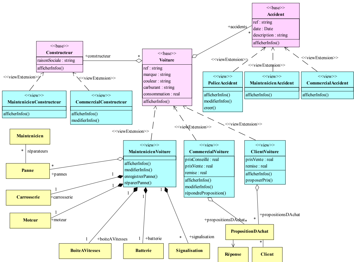
Figure 1 : Exemple de modèle VUML “Concessionnaire de voitures”
