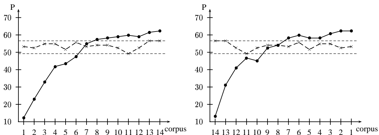
FIG. 3 – Précision des traductions obtenues pour la direction anglais-français (paramètres pour les courbes en pointillés : IM en langue source, IM3 en langue cible et jaccard pondéré)
