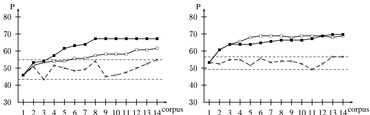
FIG. 4 – Précision des traductions obtenues par combinaison de résultats pour les directions français-anglais à gauche et anglais-français à droite (moyennes arithmétique □ et harmonique ■)
