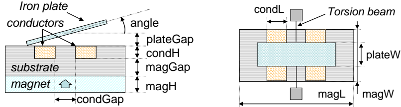
Fig. 7 – geometrical design parameters
