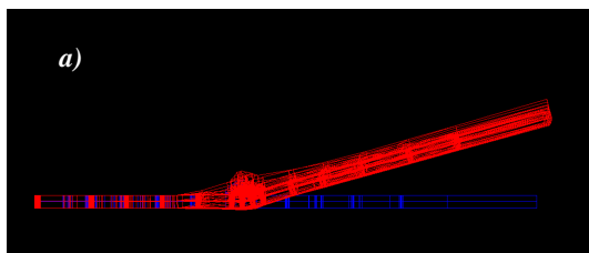
FIG 5. Déformée (rouge, amplifiés 30 fois) avant débridage (a) (vue le long du cordon) et après débridage (b) (en bleu le maillage non déformé)
