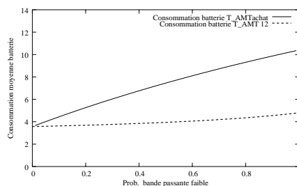
Figure 3. Consommation de batterie vs bande passante (deux T_{AMT} ).
