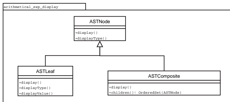
Figure 5. le modèle décrivant l’affichage d’un arbre
