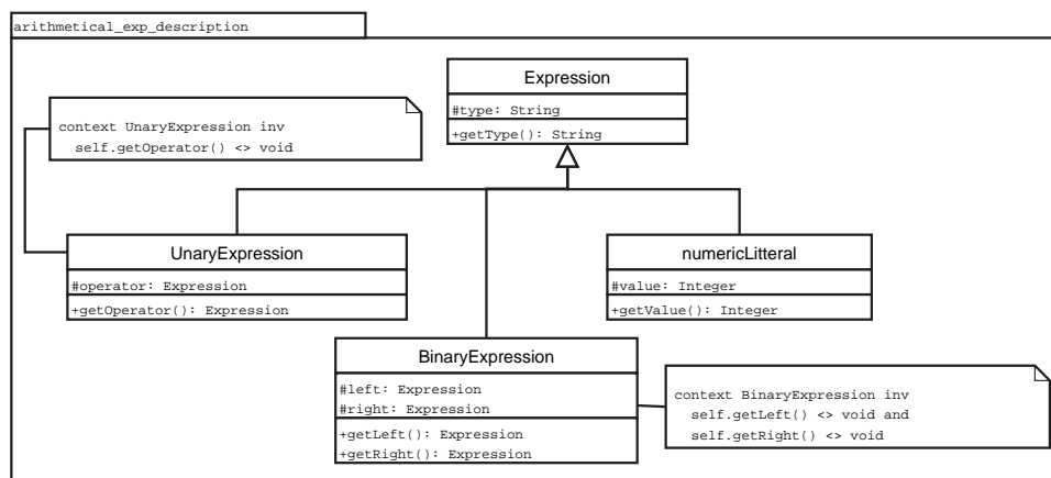
Figure 7. le modèle décrivant l'arbre des expressions arithmétiques
