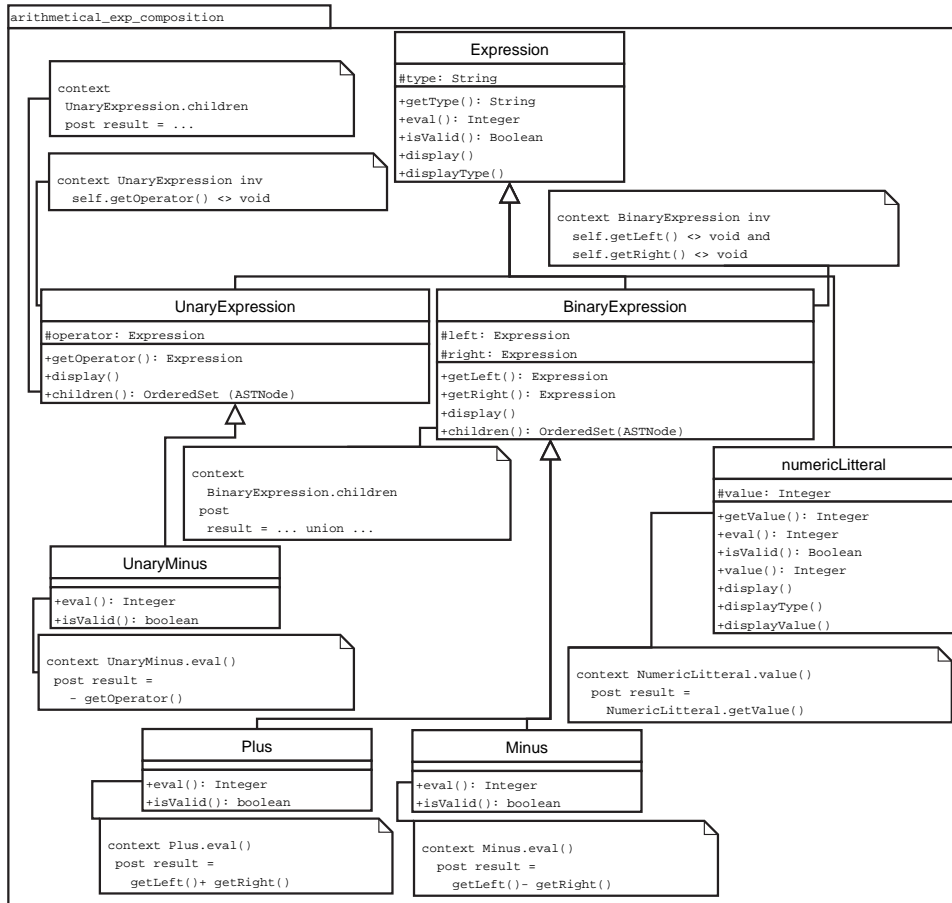
Figure 11. Résultat de la deuxième composition
