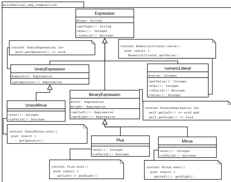
Figure 10. Résultat de la première composition
