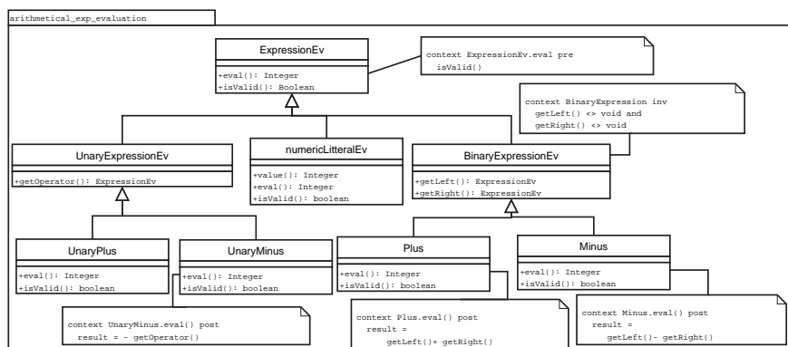
Figure 3. le modèle décrivant l'évaluation des expressions arithmétiques
