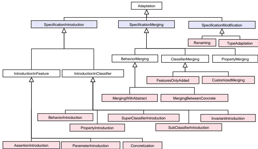
Figure 2. la hiérarchie des adaptations sur les modèles
