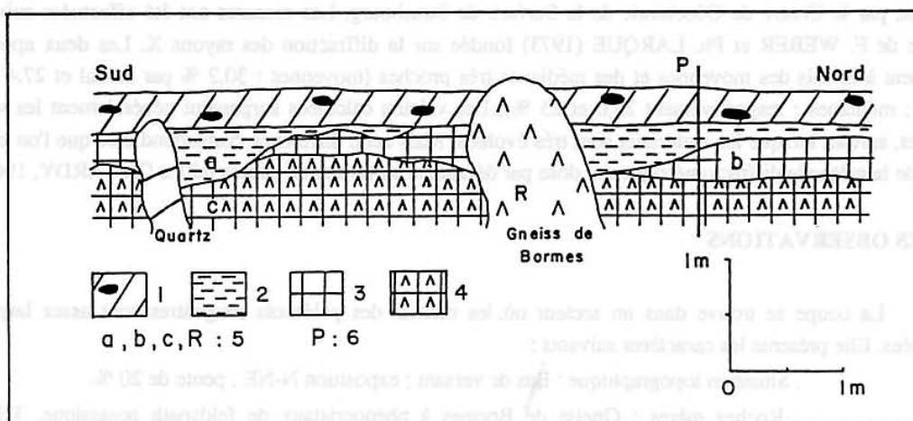
Figure 2 - Présentation de la coupe.
