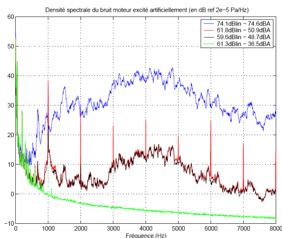
FIG. 2 – Conditionnement du bruit émis par le moteur excité artificiellement par le signal alimentant le pot vibrant et par le signal boîtier papillon (contact moteur établi). En bleu : spectre de bruit total. En rouge : spectre conditionné par le signal du pot vibrant. En noir : spectre conditionné par le signal pot et le signal boîtier papillon. En vert : bruit de fond.
