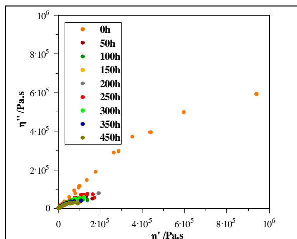
Fig. 2 : Diagramme Cole-Cole représentant l'évolution de la viscosité du mélange PLA – peuplier A 0,25 mm rétifé au cours des irradiations
