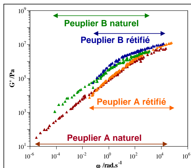
Fig. 1 : Courbes maîtresses des mélanges PLA – peuplier A et B, naturel et réifié pour la température 180°C.
