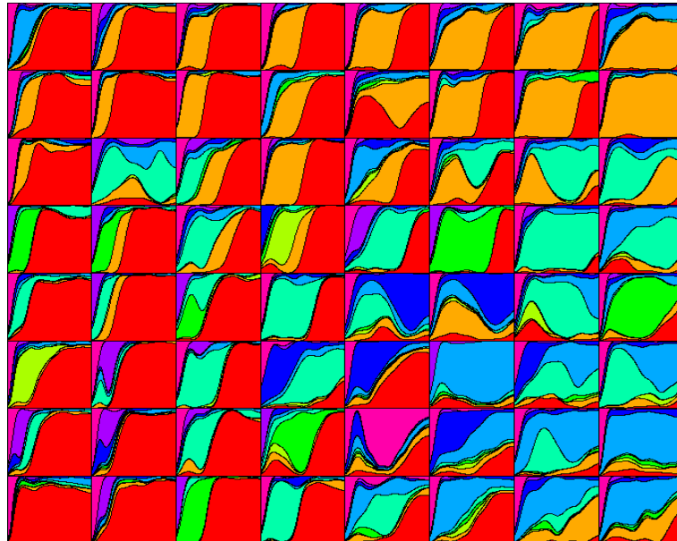
Fig. 2. SOM 8x8
