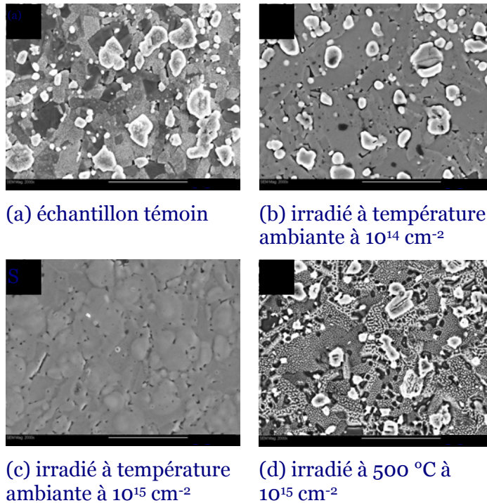
Figure 1 : Images MEB, grossissement \times 2000
