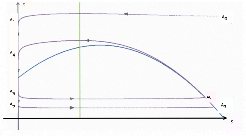
FIG. 2 – Le cycle limite du système (5)
