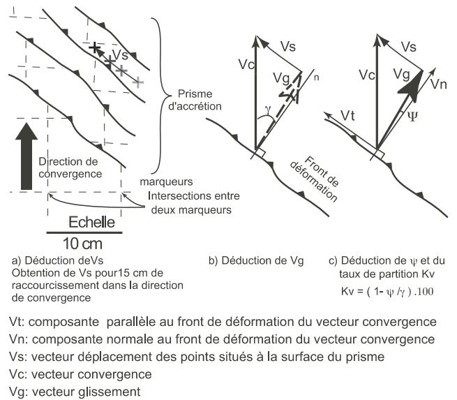
FIG. 2. – Procedure to determine the slip vector Vg, its angle of obliquity \psi with the perpendicular to the deformation front, and the partition rate Kv (%). FIG. 2. – Procédure de détermination du vecteur glissement Vg de son angle d’obliquité \psi avec la normale au front de déformation ainsi que du taux de partition Kv (%).
