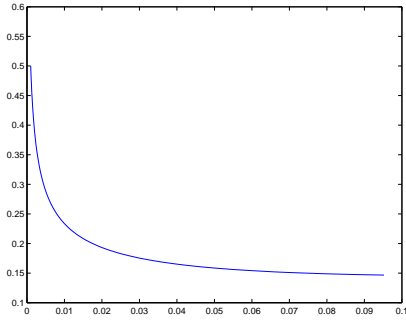
Fig. 17. \sqrt{\varepsilon} \log \varepsilon \|u^\varepsilon\|_{L^2(O_\varepsilon)} = f(\varepsilon)
