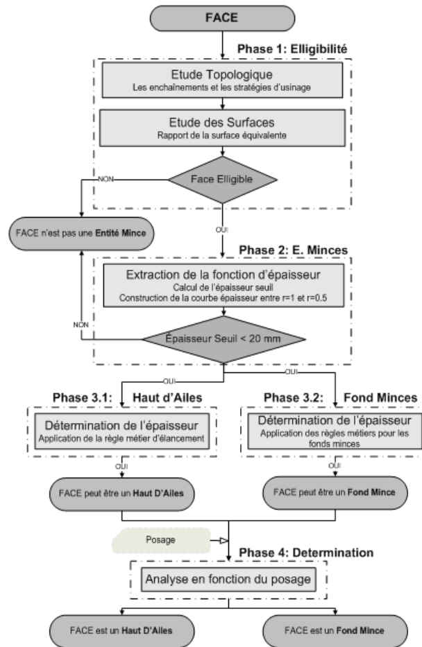
Figure 4. Algorithme de détection des hauts d'aile et fonds mince
