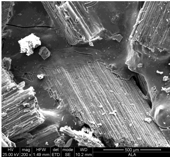
Fig. 4 : Analyse micro structurelle des Composites agrolisés à base d'anas de lin (grossissement : 200).
