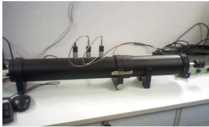
Fig. 8 : Tube de Kundt
