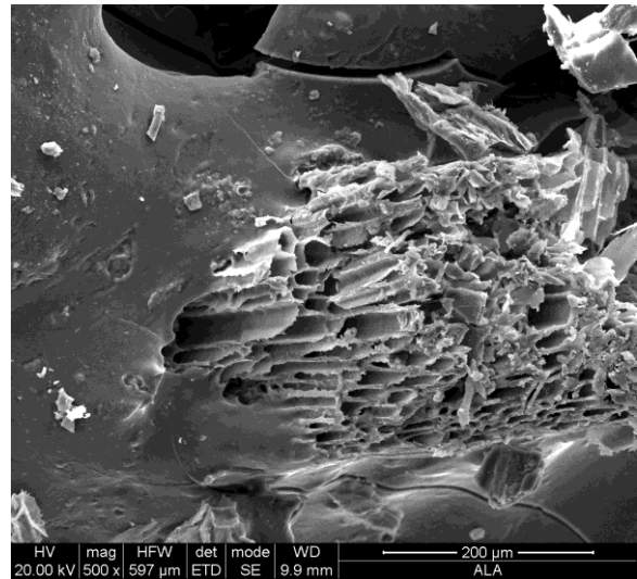
Fig. 5 : Analyse microstructurelle de la structure des anas présents dans un composite agrolisé (grossissement : 500).
