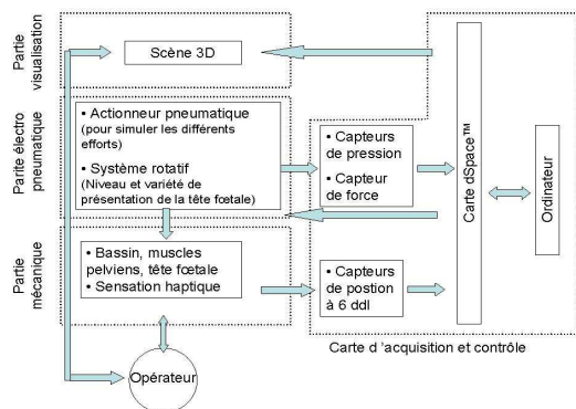
Fig. 1. Schéma de principe du simulateur BirthSIM
