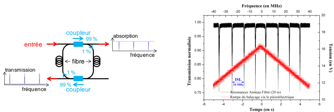
(a) Schéma de principe de l'anneau de fibre. (b) Mesure de l'ISL en "scan" direct de l'anneau.
