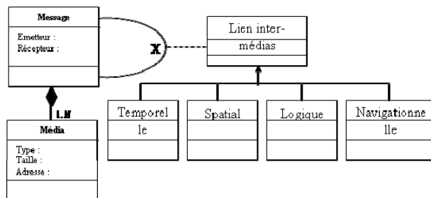
Figure 3. Diagramme de classe représentant les différents liens entre média
