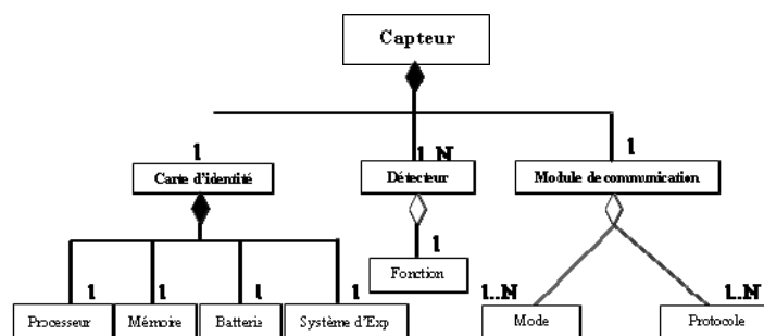
Figure 1. Diagramme de classe d'un capteur
