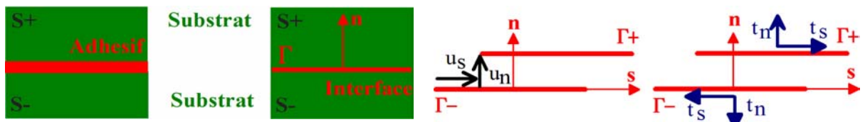
(a) Modèle d'interface
