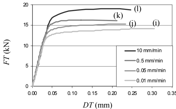
(c) Comportement dans la direction tangentielle pour des essais de traction-cisaillement ( \gamma = 45^\circ )
