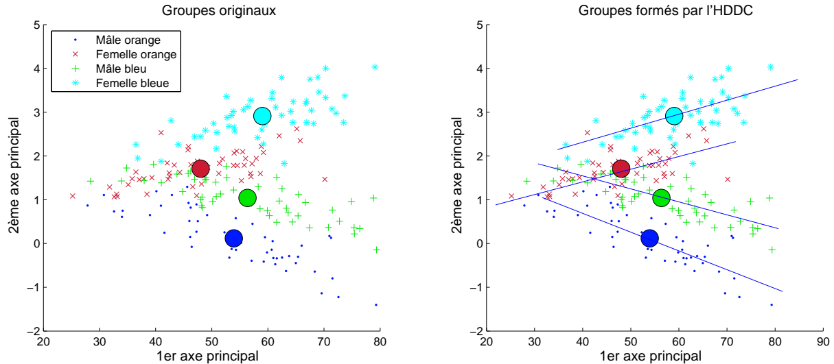
FIG. 5 – Classification non supervisée grâce à l’HDDC des données « Crabes » : à gauche, données projetées sur le premier plan principal et, à droite, segmentation obtenue avec le modèle [a_i b_i Q_i d_i] de l’HDDC ainsi que les sous-espaces spécifiques estimés (lignes bleues).
