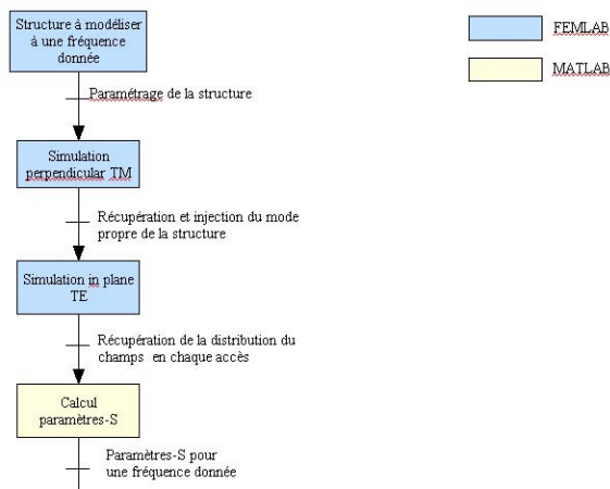
Figure.1 : algorithme de calcul des paramètres-S d'un composant optique
