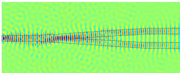
Figure.3b : Propagation d'un champ unitaire dans la structure
