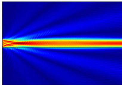
Figure.2: Détermination du mode propre d'un guide.
