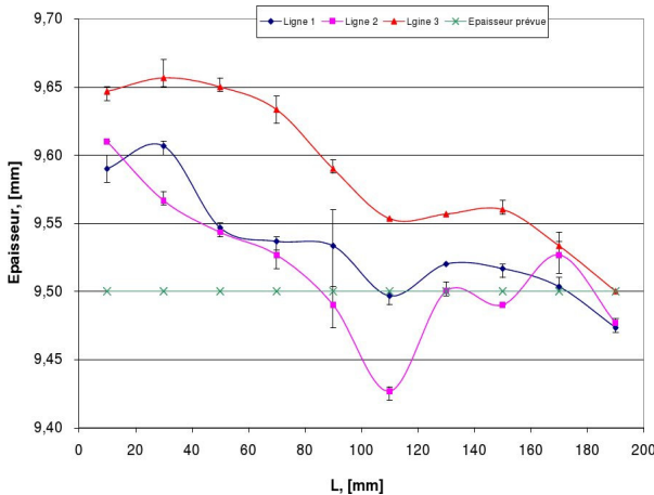
Fig. 3.4. Variation d'épaisseur de la pièce 2, épaisseur considérée entre Plan 2 et Plan 4.
