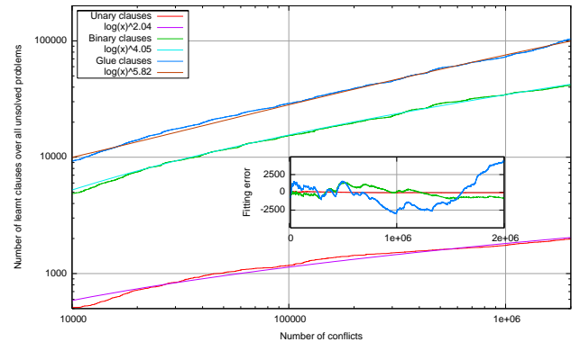
FIG. 5 – Nombre cumulé de clauses apprises (unaires, binaires, glues) produites durant la recherche, restreinte aux problèmes non résolus. En petit, nous avons représenté l'erreur de "fitting".
