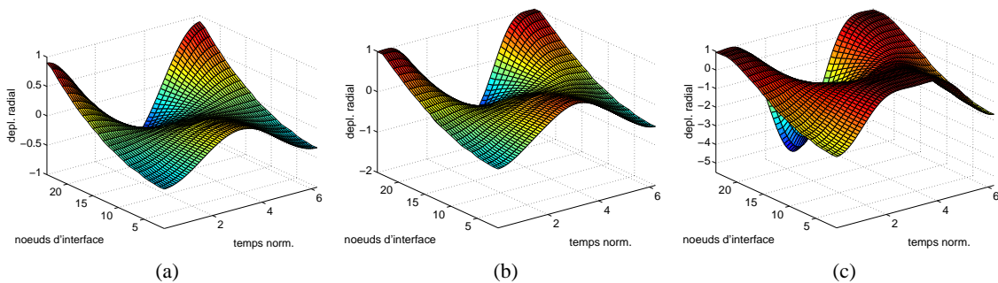
Figure 3: Déplacements radiaux à l'interface pour trois valeurs de l'amplitude modale : (a) 5.7, (b) 9.3 et (c) 31.3. Le contact a lieu pour une amplitude égale à 1.
