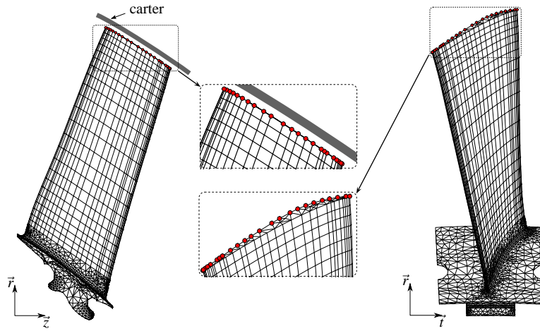
Figure 1: Modèle de l'aube et détails de l'interface de contact
