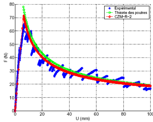
Fig. 10. Comparaison des courbes force-déplacement pour une éprouvette DCB.
