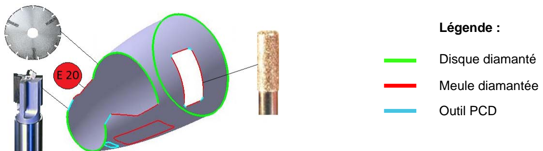
Fig. 5. Résultat obtenu suite à l'analyse locale de la pointe avant d'avion.
