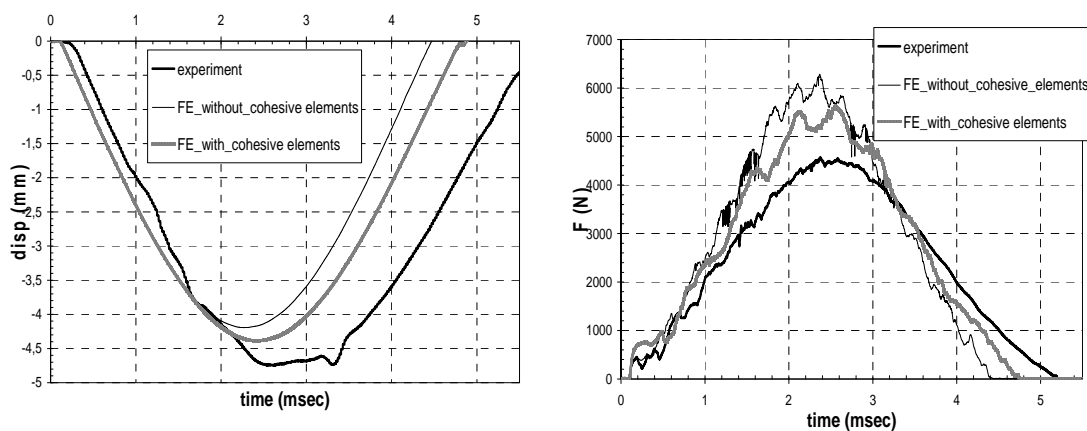
Fig. 9. Comparaison essai/calcul : (a) déplacement max-temps (b) effort max-temps
