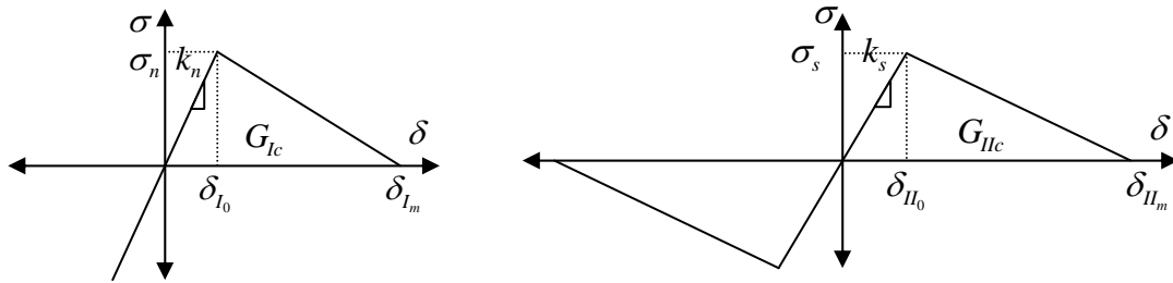
Fig. 1. Comportement du modèle cohésif utilisé
