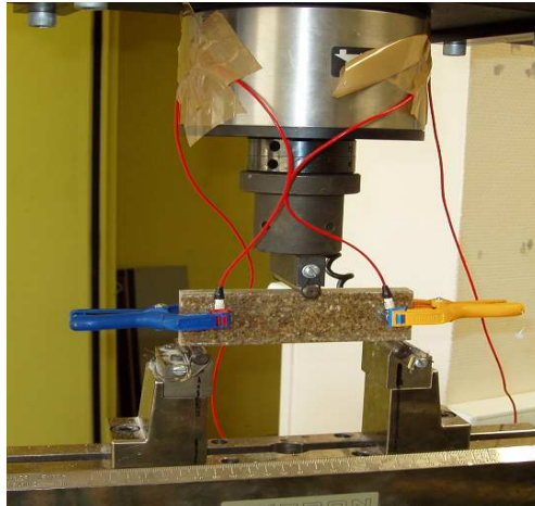
Fig. 1. Dispositif expérimental.
