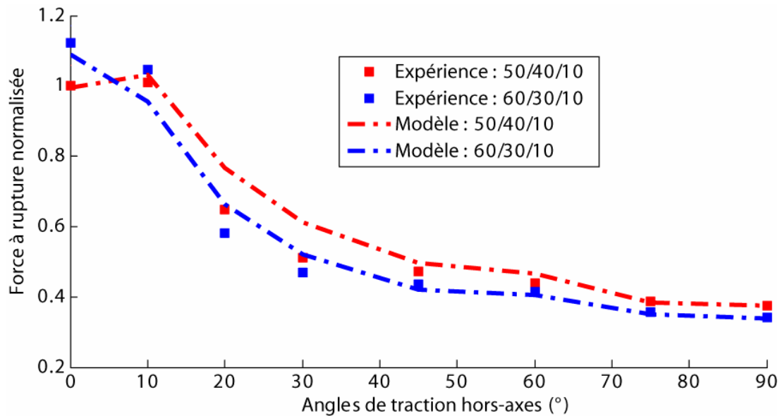
Fig. 8. Comparisons essais/calculs sur des plaques perforées en T700/M21 présentant différents empilements soumises à des efforts de traction uniaxiale hors-axe.
